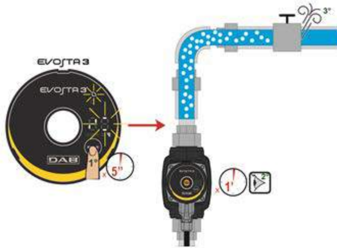
Abb. 9: Automatische Pumpenentlüftung
