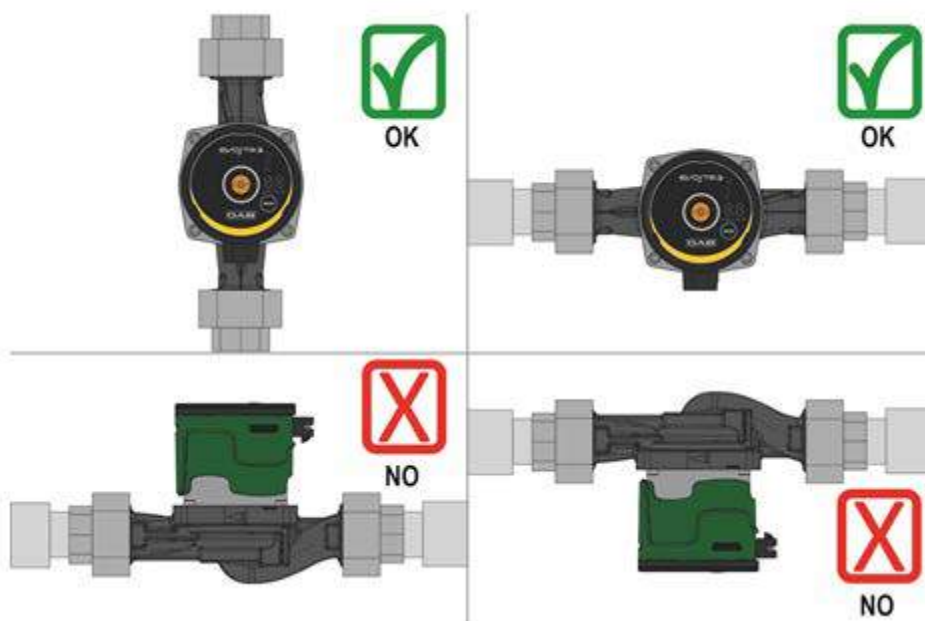
Afbeelding 3: montagepositie
