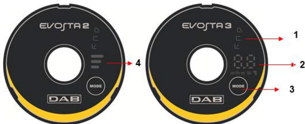
Figura 10: Visor
